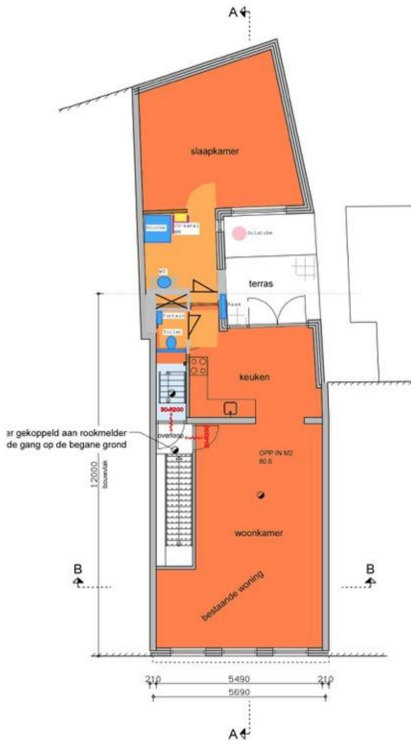
1e VERDIEPING
